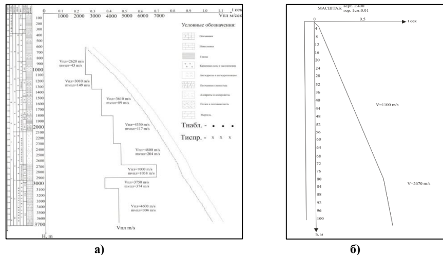
Рис.2. Денгизкуль скв.№1П а) – ВСП, б) – МСК
